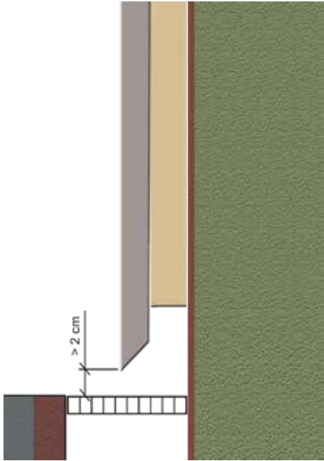
S-Punkt 4: Mindestens 2 cm bei Metallrosten. Die Roste müssen zur Reinigung der darunter liegenden Rinnen herausnehmbar sein.
