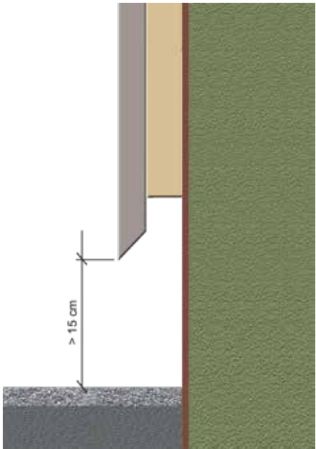
S-Punkt 3: Mindestens 15 cm bei einer mindestens 200 mm breiten Kiesschüttung (16/32 Kornschüttung).
