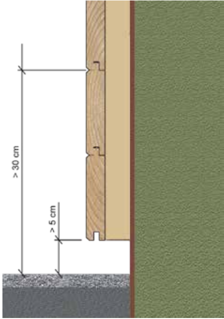
S-Punkt 2: Das breite Kiesbett (16/32 Kornschüttung) ermöglicht es, das unterste Sockelbrett bis auf 5 cm heranzuführen, zusätzlich kann das unterste Brett auch problemlos ausgetauscht werden.
