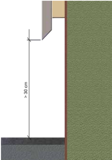
S-Punkt 1: Mindestens 30 cm bei harten Untergründen (z.B. Betonpflaster) und glatten Böden bis 50 cm.
